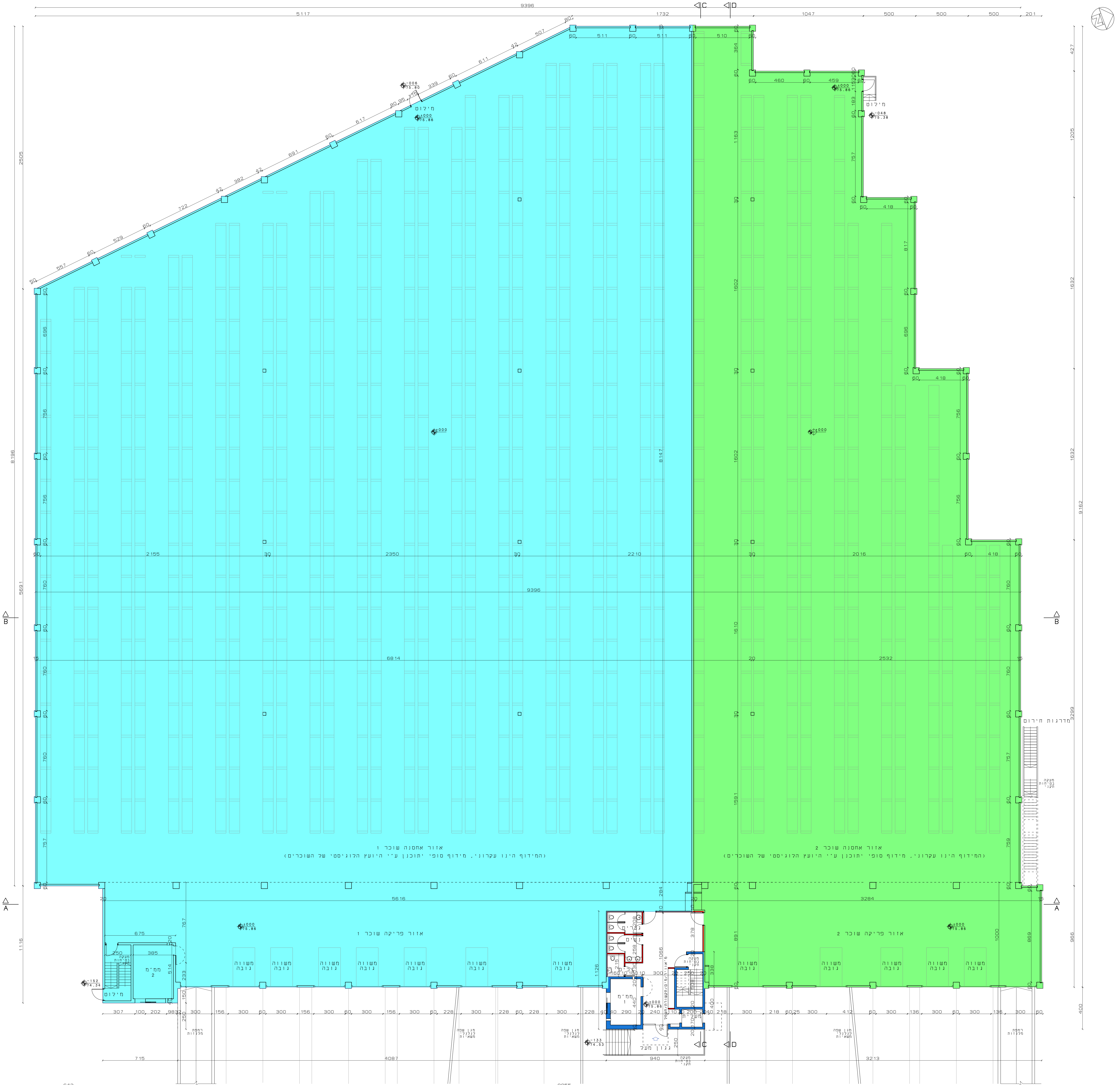
תכנית מפלס ±000 קני"מ 1:125
